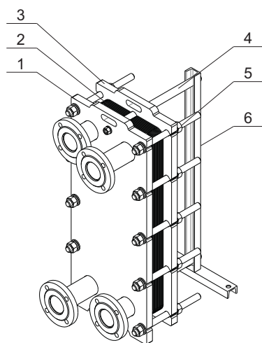
Рис. 1 - Теплообменник в сборе
