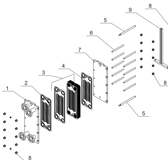
Рис. 2 - Детализовка теплообменника
